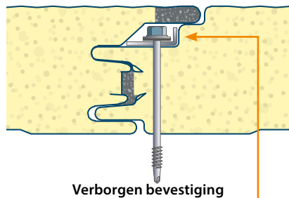
Verborgene bevestiging
