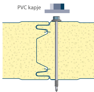
Zichtbare bevestiging driedubbele sluiting
